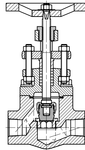
NPT SUIVANT/ acc. to ANSI B1.20.1
