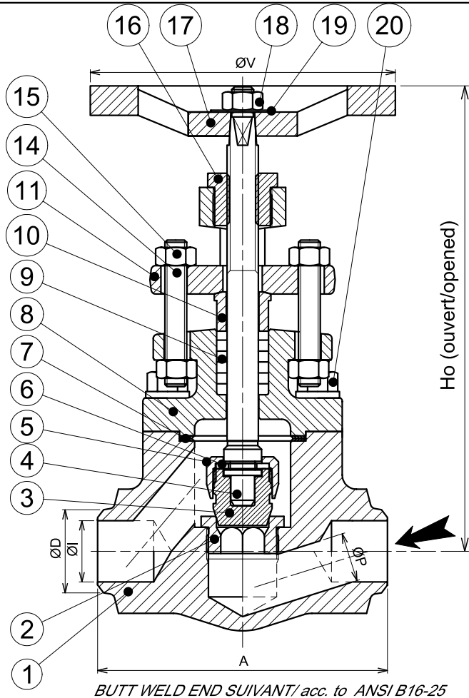
BUTT WELD END SUIVANT/ acc. to ANSI B16-25
